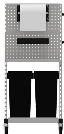
Station hygiénique « Smart-Clean » 2 parois arrières perforées 1 tablette amovible 1 support pour rouleau de papier et porte-bouteilles 3 poubelles de 60 litres
